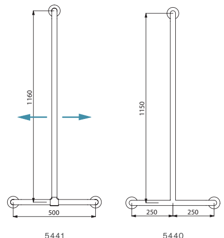
Position der Brausestange bei Montage einstellbar (Art. 5441)
