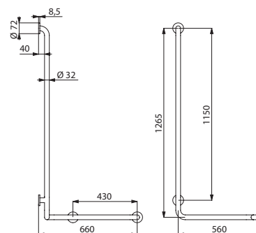
Rechte Ausführung - 5100D
