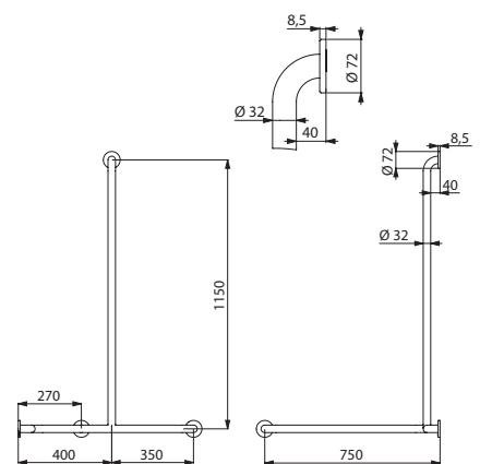
Rechte Ausführung - 5481D
