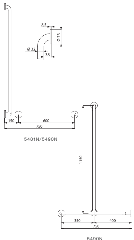
Position der Brausestange bei Montage nach links oder rechts einstellbar (Art. 5481N)
