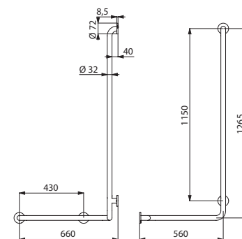
Linke Ausführung - 5100G
