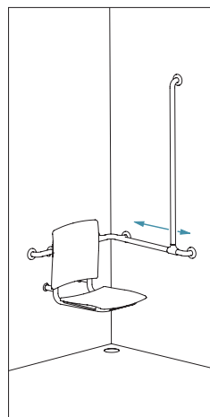
Position der Brausestange bei Montage nach links oder rechts einstellbar (Art. 5481N)
