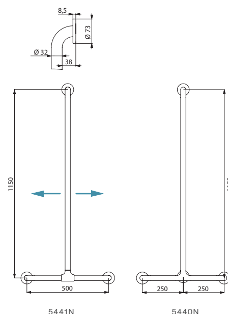
Position der Brausestange bei Montage einstellbar (Art. 5441N)
