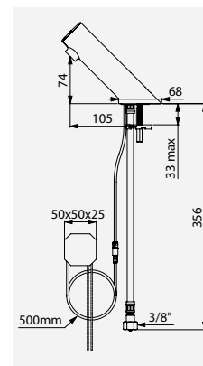
Ventil TEMPOMATIC 5 für Netzbetrieb Art. DELABIE: 449100
