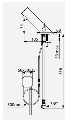
Mischbatterie TEMPOMATIC 5 für Netzbetrieb Art. DELABIE: 499100
